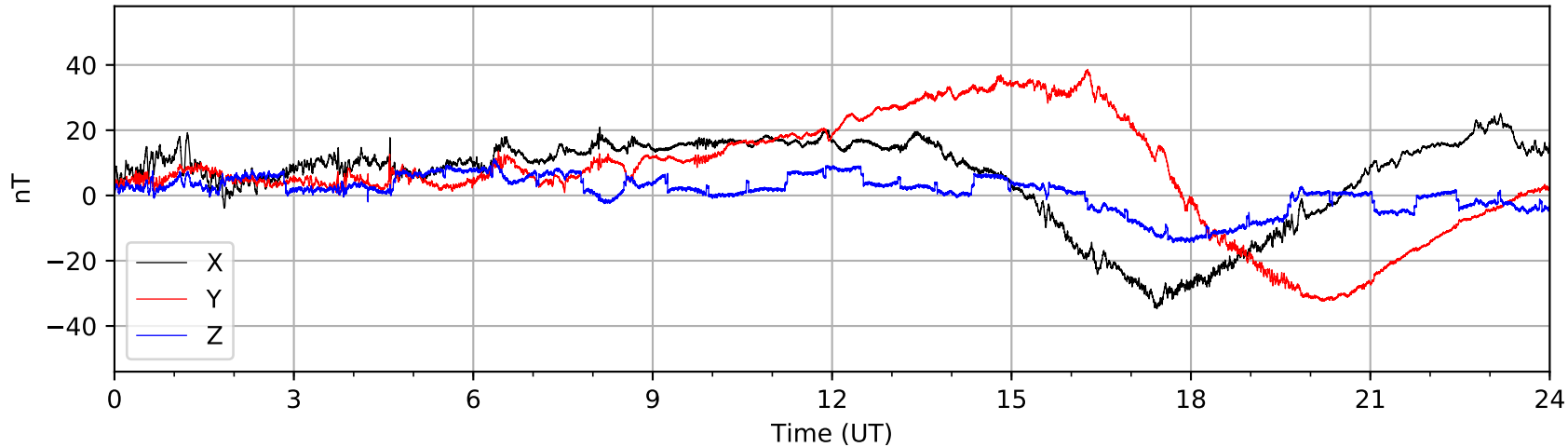
Bartington MAG03 (AUGO) 2021-08-22
