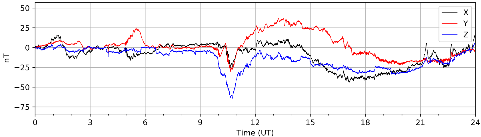
Bartington MAG03 (AUGO) 2021-08-17
