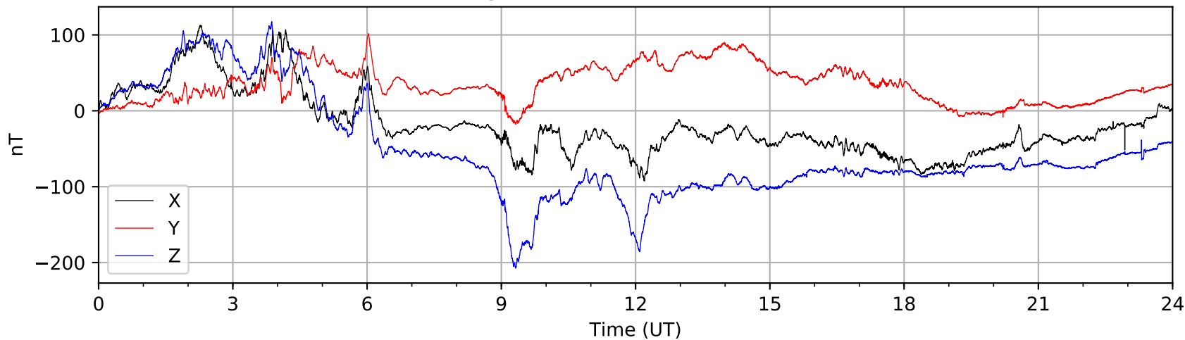
Bartington MAG03 (AUGO) 2021-08-07
