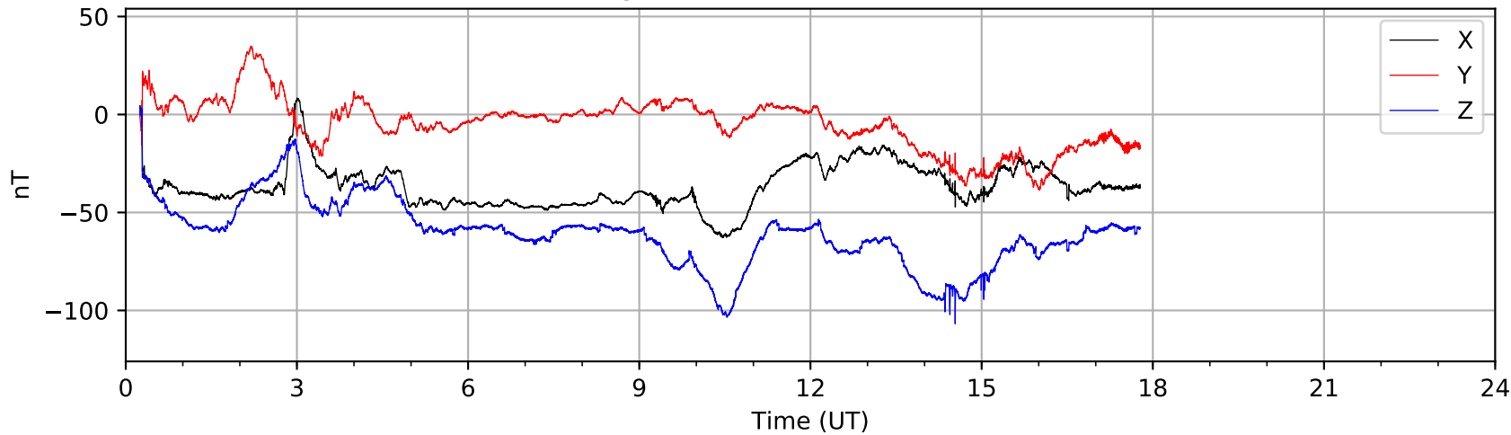
Bartington MAG03 (AUGO) 2021-07-21
