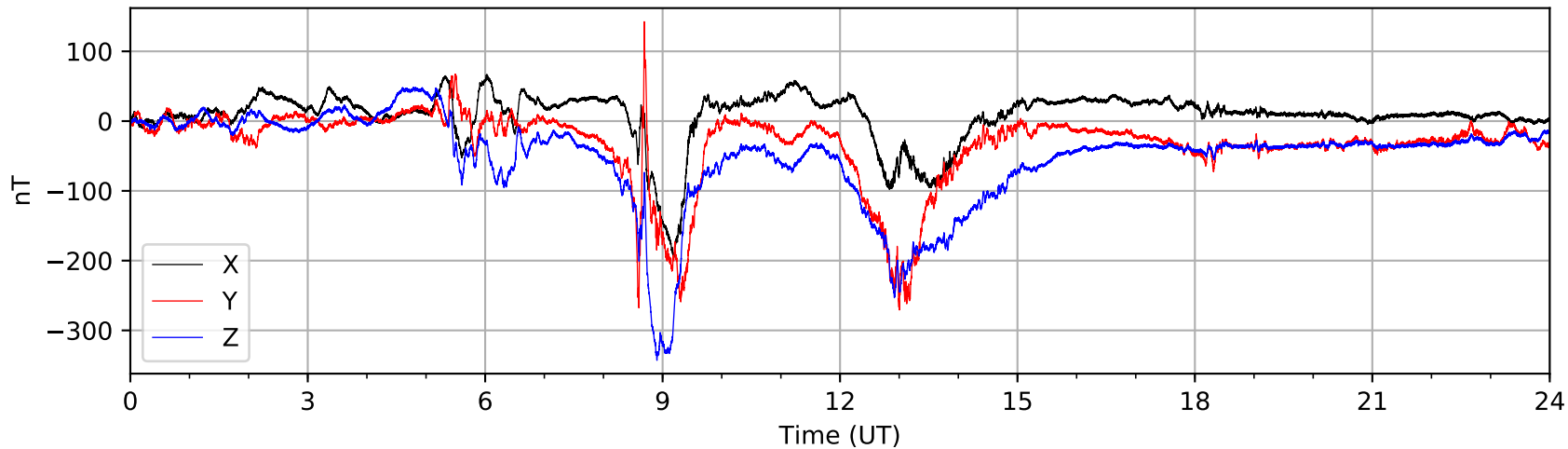
Bartington MAG03 (AUGO) 2021-02-21
