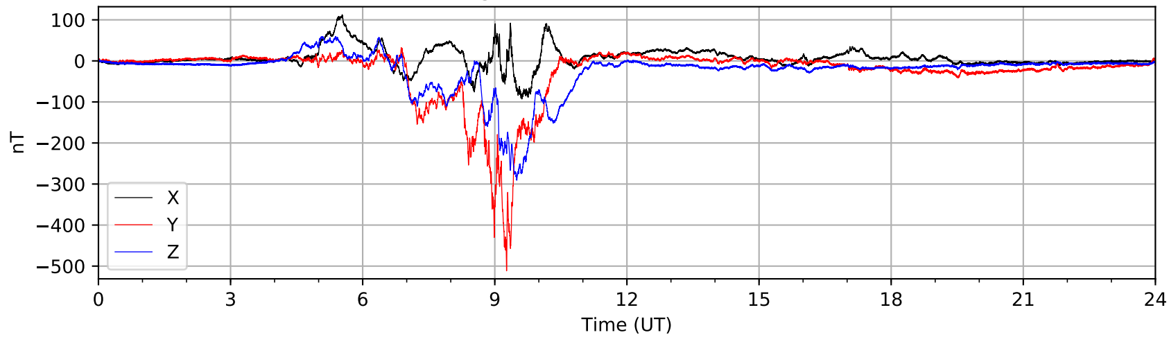
Bartington MAG03 (AUGO) 2021-02-16
