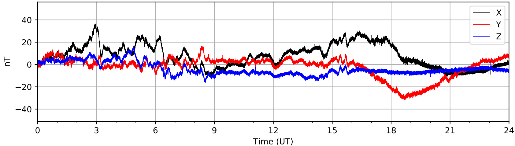
Bartington MAG03 (AUGO) 2021-02-14
