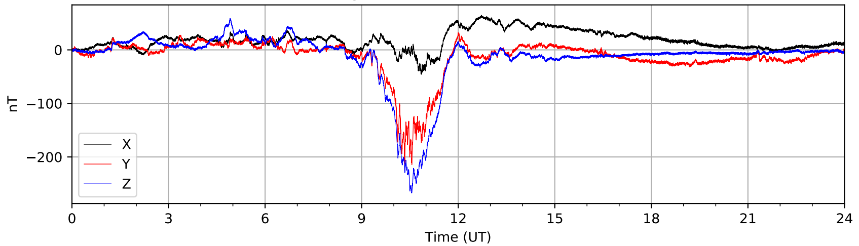
Bartington MAG03 (AUGO) 2021-02-13
