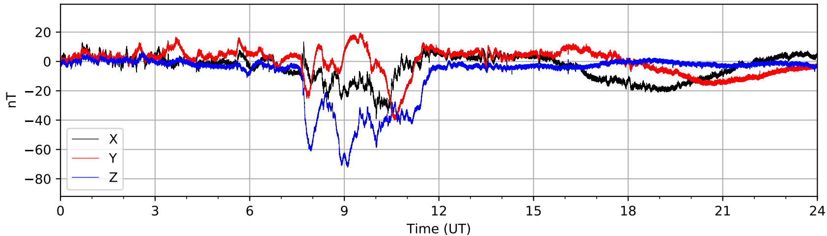
Bartington MAG03 (AUGO) 2021-02-09
