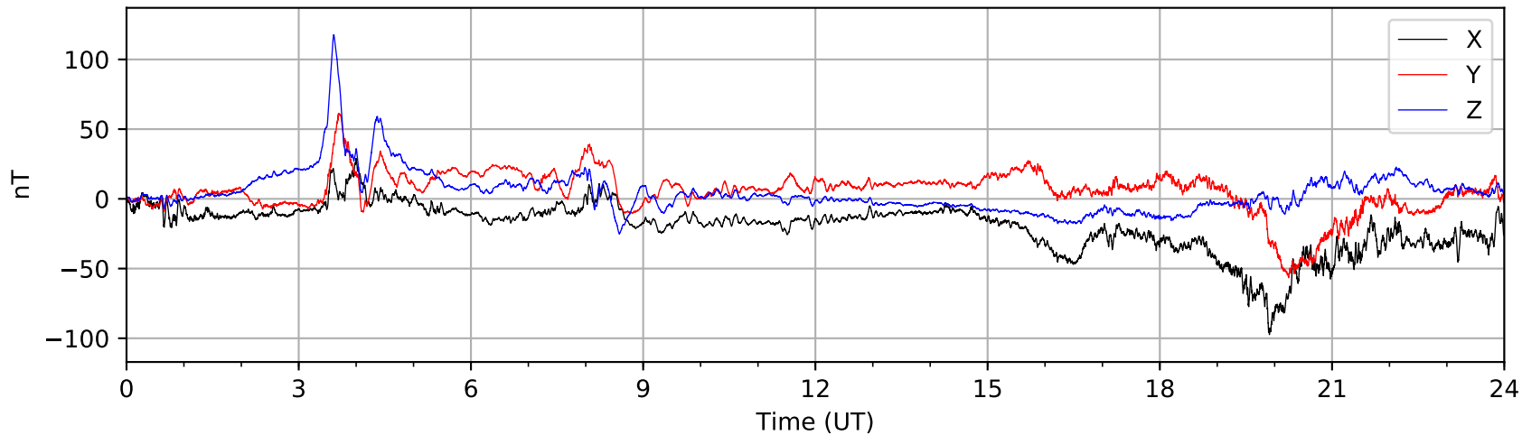
Bartington MAG03 (AUGO) 2021-02-03
