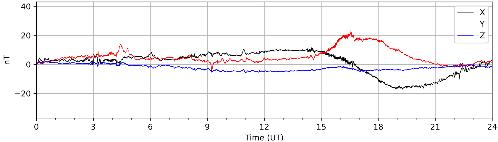
Bartington MAG03 (AUGO) 2021-01-21
