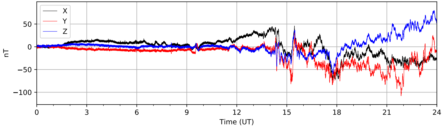
Bartington MAG03 (AUGO) 2021-01-11
