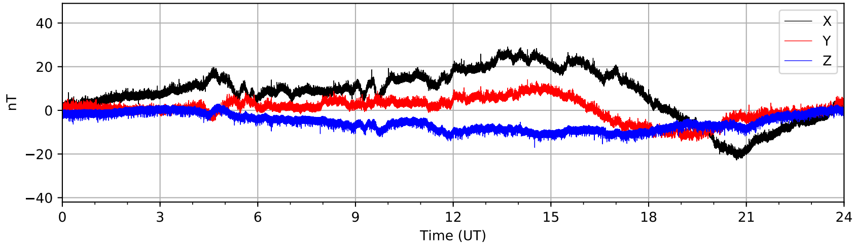
Bartington MAG03 (AUGO) 2021-01-10
