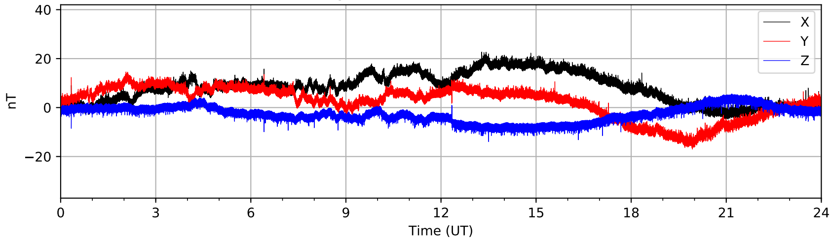
Bartington MAG03 (AUGO) 2021-01-09
