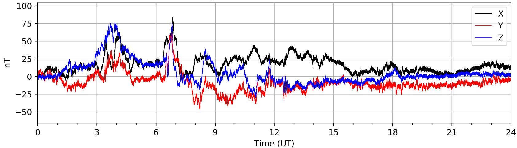
Bartington MAG03 (AUGO) 2021-01-06
