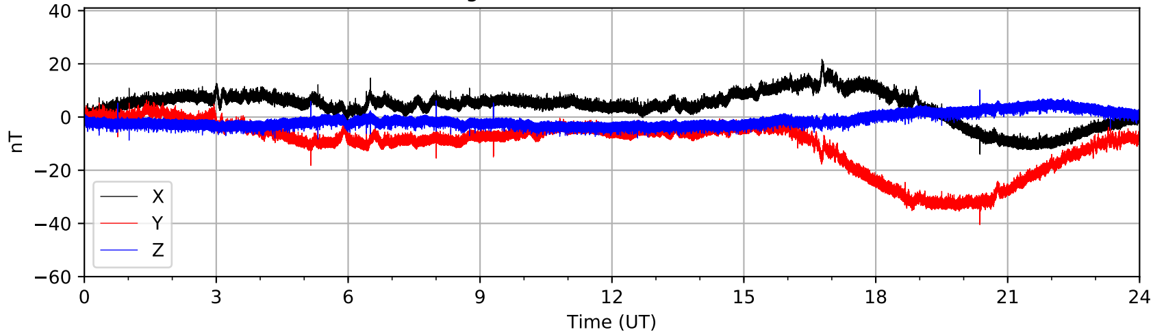
Bartington MAG03 (AUGO) 2021-01-03
