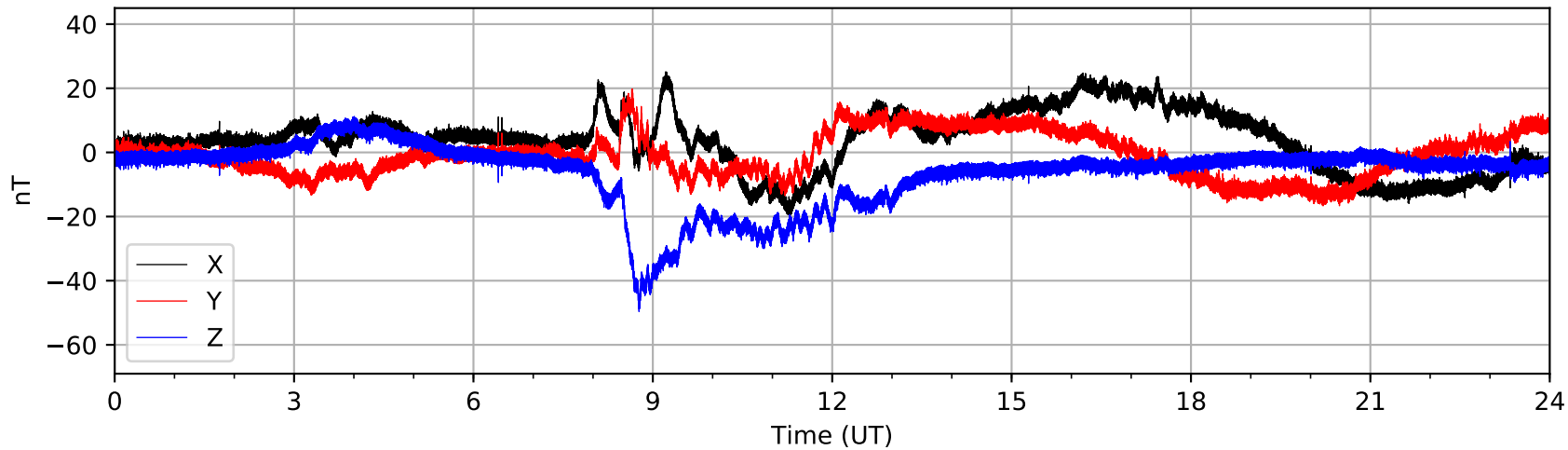
Bartington MAG03 (AUGO) 2020-12-08
