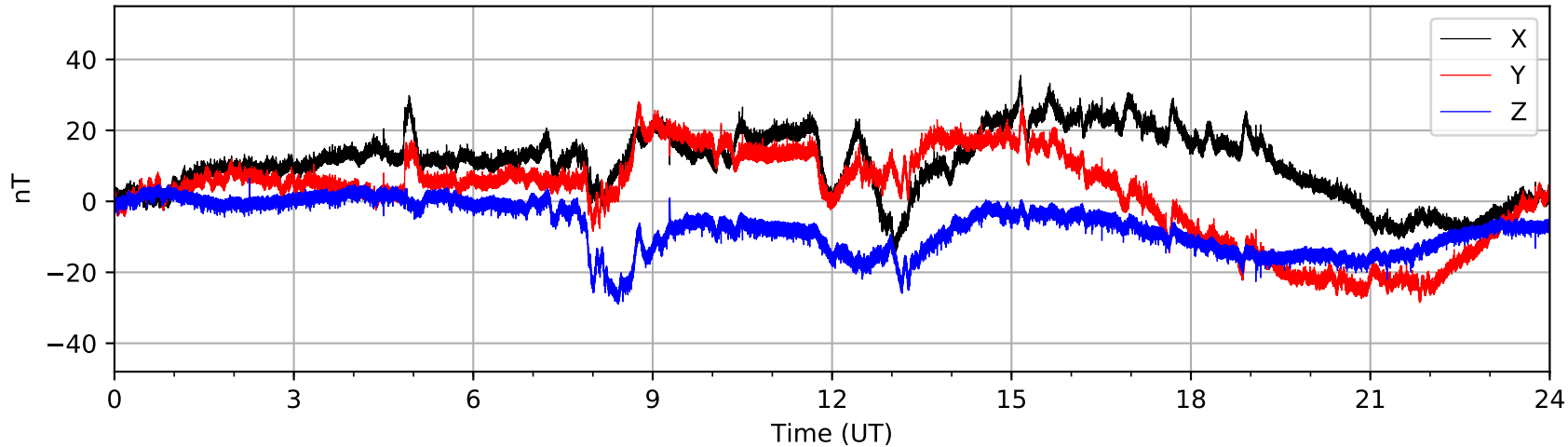
Bartington MAG03 (AUGO) 2020-12-06
