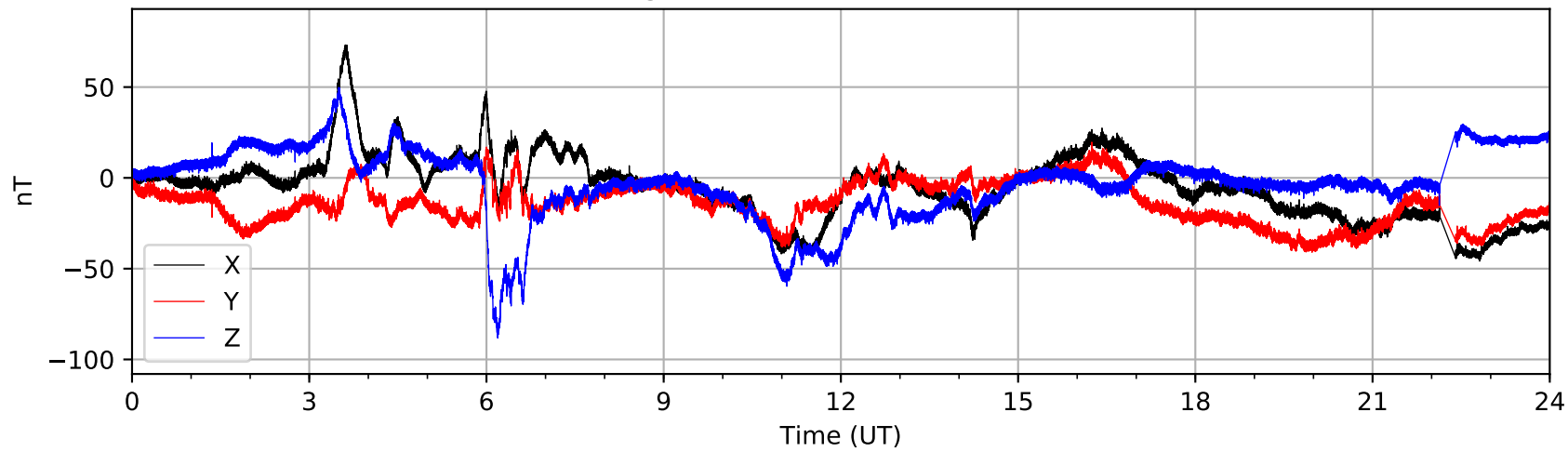
Bartington MAG03 (AUGO) 2020-11-28
