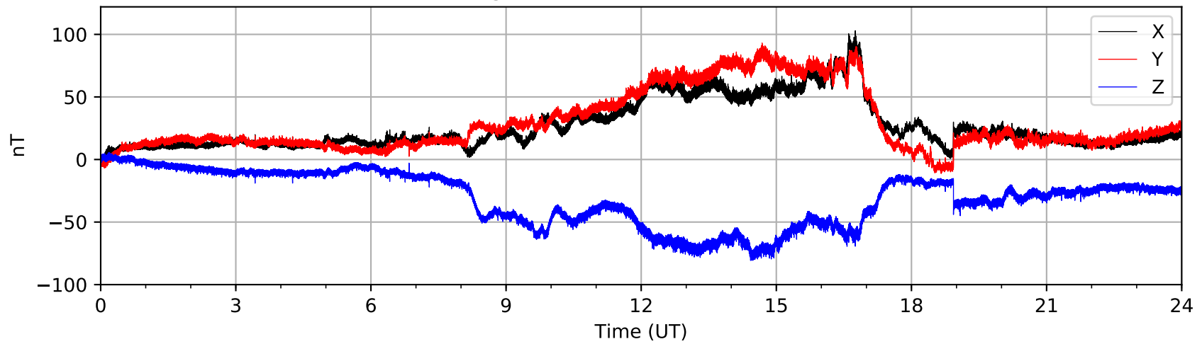
Bartington MAG03 (AUGO) 2020-11-26
