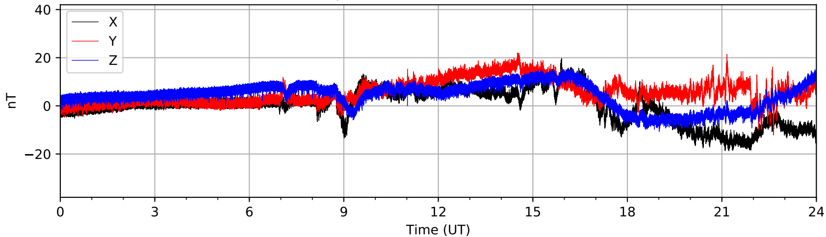
Bartington MAG03 (AUGO) 2020-11-11
