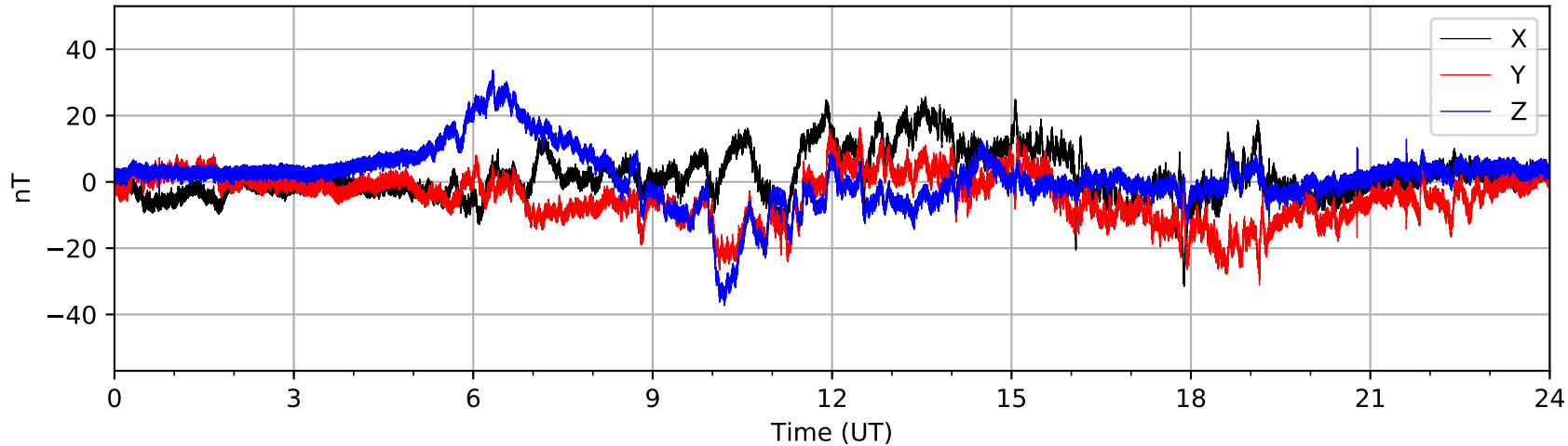
Bartington MAG03 (AUGO) 2020-11-06
