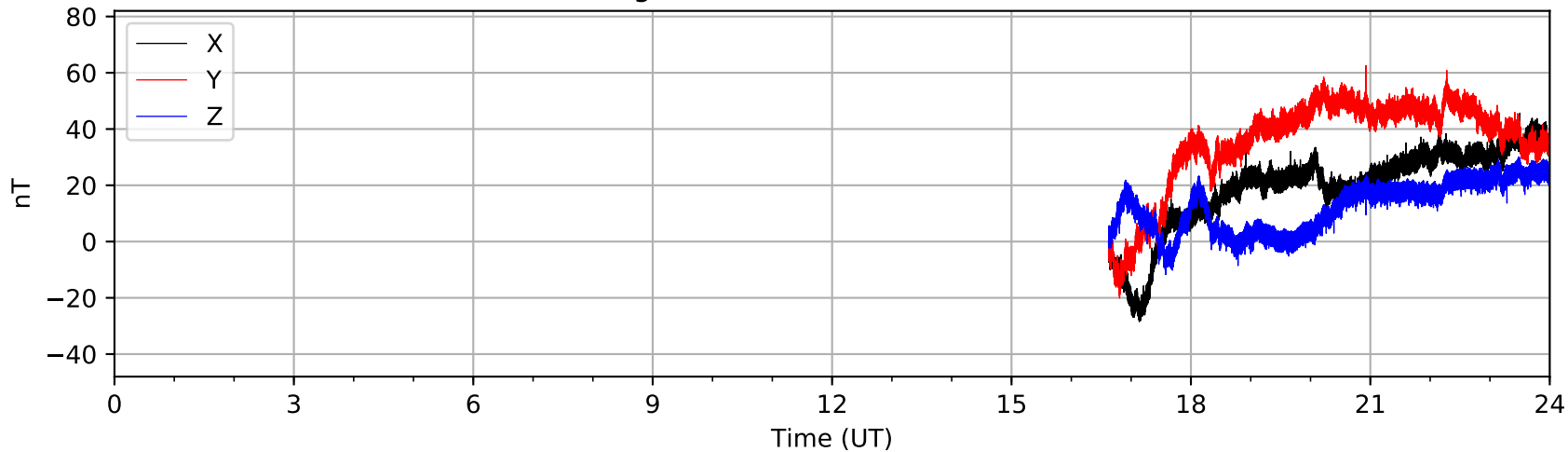
Bartington MAG03 (AUGO) 2020-10-29
