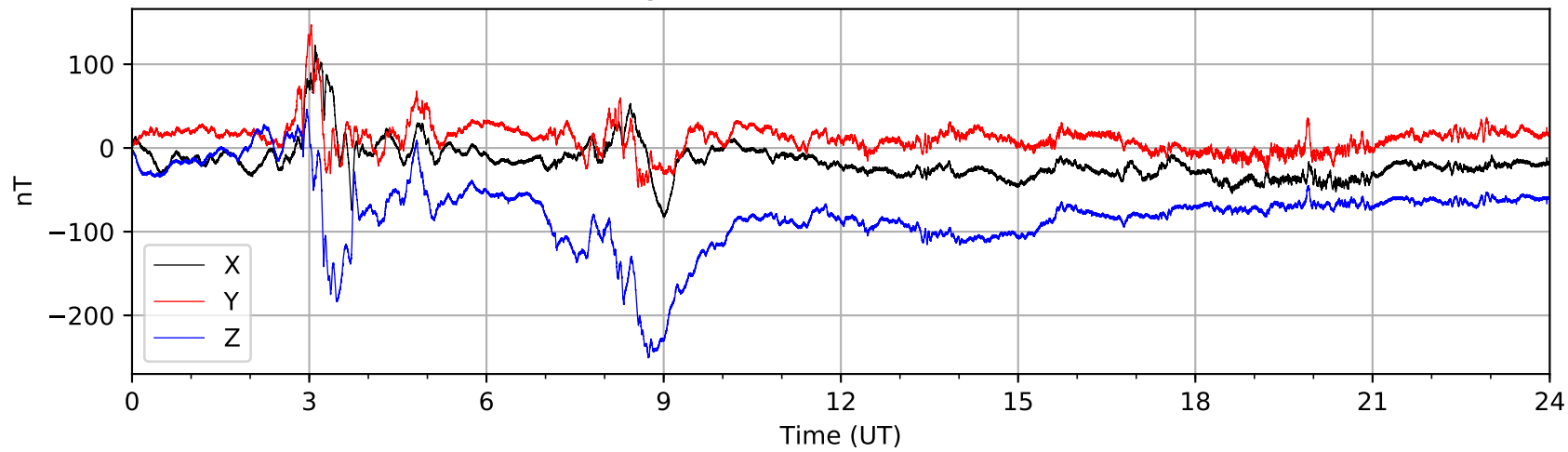
Bartington MAG03 (AUGO) 2020-10-24
