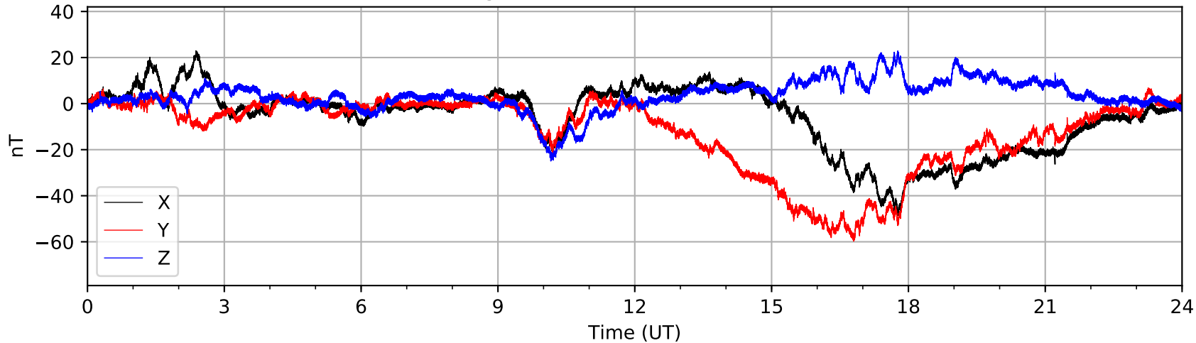
Bartington MAG03 (AUGO) 2020-10-04
